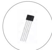
TO94-4L(VK) 5.22*3.65*1.56
