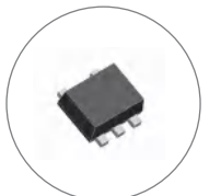
SOT553-5L(SN) 1.6*1.2*0.6
